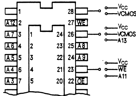
Bild 3. Verschiedene Speicher benötigen unterschiedliche Signale an bestimmten Anschlußpins
