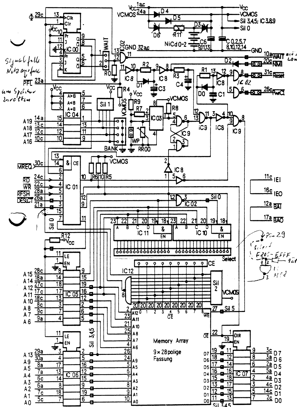
Bild 2. Die Gesamtschaltung der Speicherkarte
