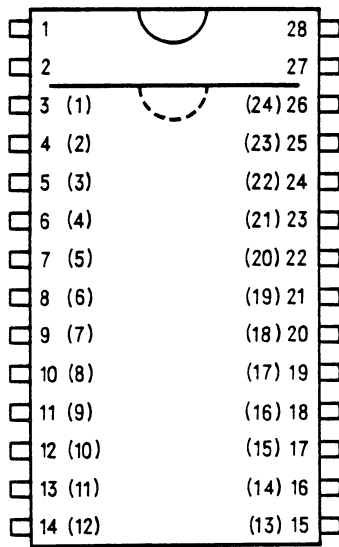
Bild 1. Die Pinbelegungen von unterschiedlichen Speichern, die in das Byte-wide-Konzept passen
