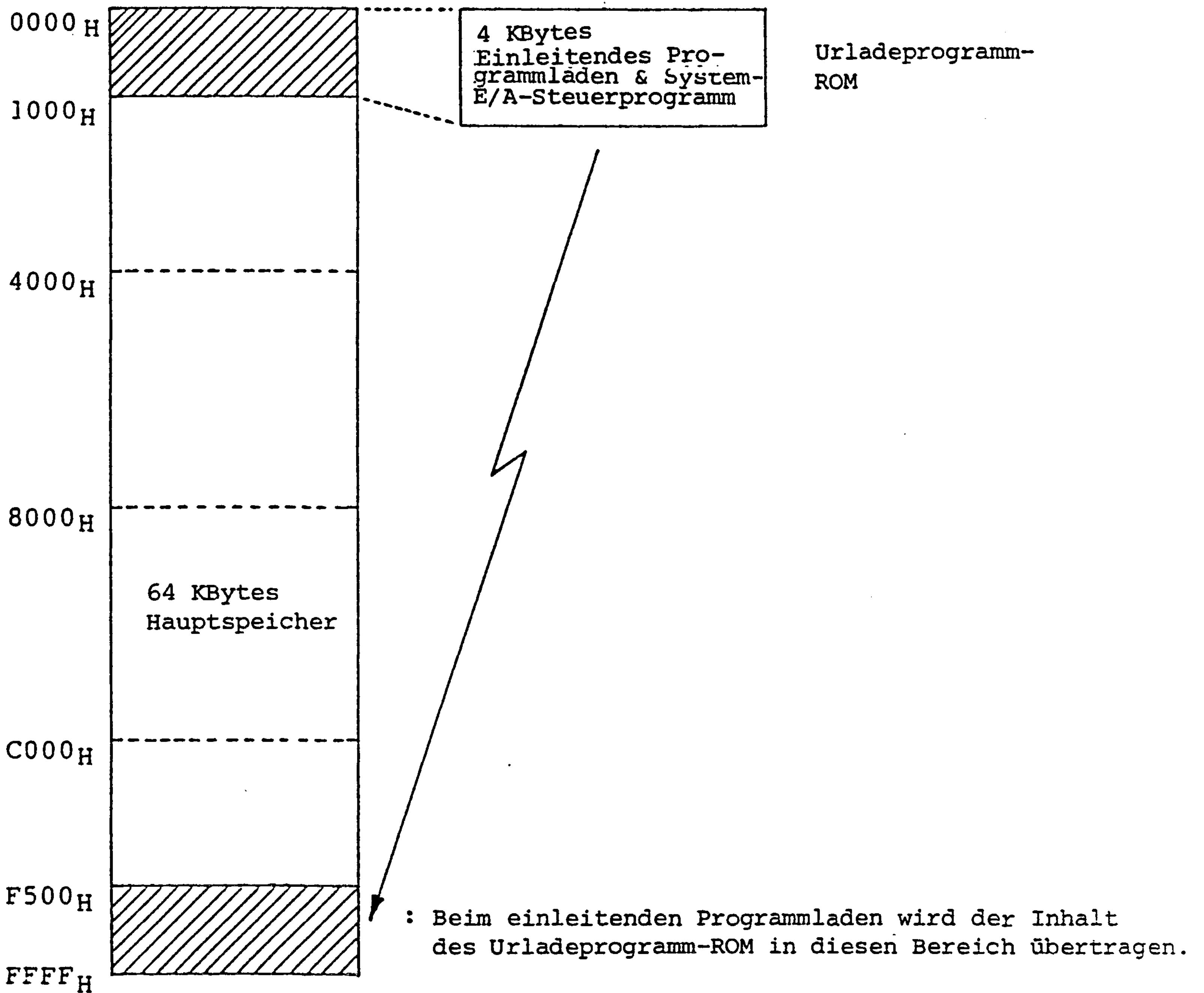
Abb. 15: Speicherzuordnung
