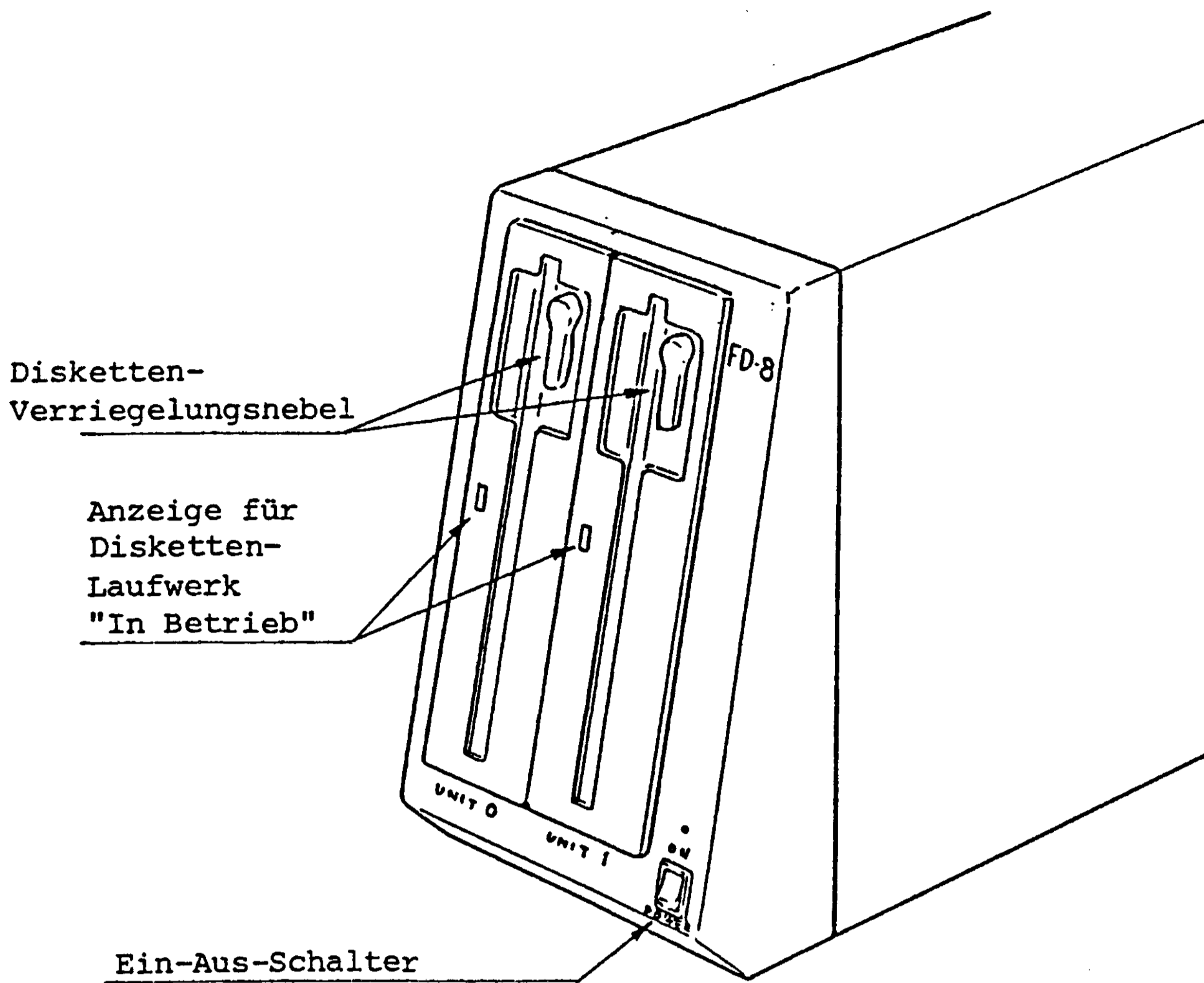
Abb. 11: Floppy-Disketten-Laufwerk FD-8
