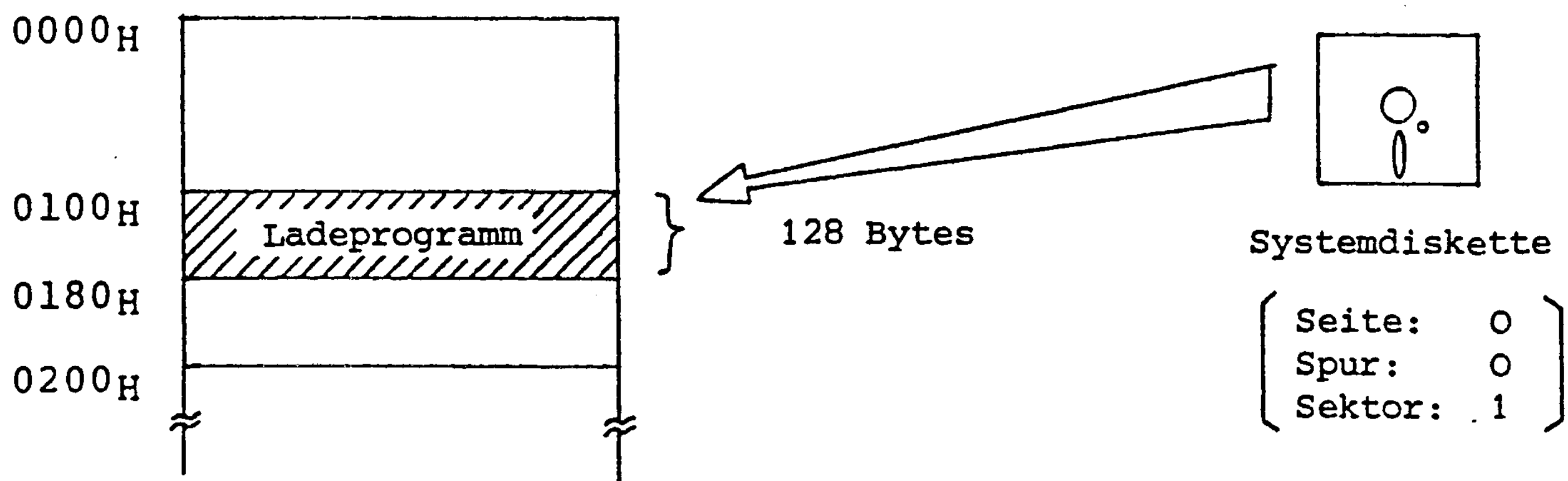
Abb. 17: Ladeprogrammzuordnung
