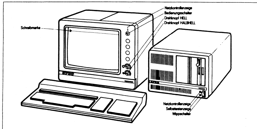
Bild 1.1: Arbeitsplatz-Computer TRANSDATA 9780
