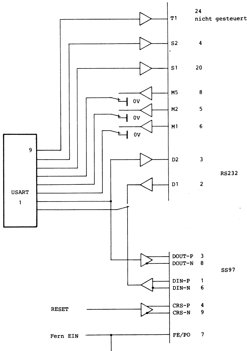
Funktionsbild SS97 / RS232
