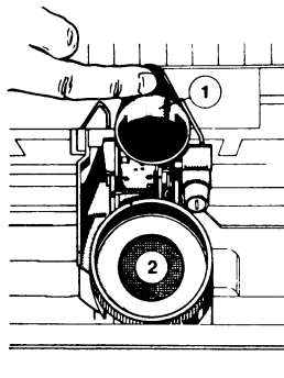
Bild 9/1 Tintendruckkopf
