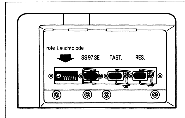
Bild 12.1: Bildschirm von hinten
