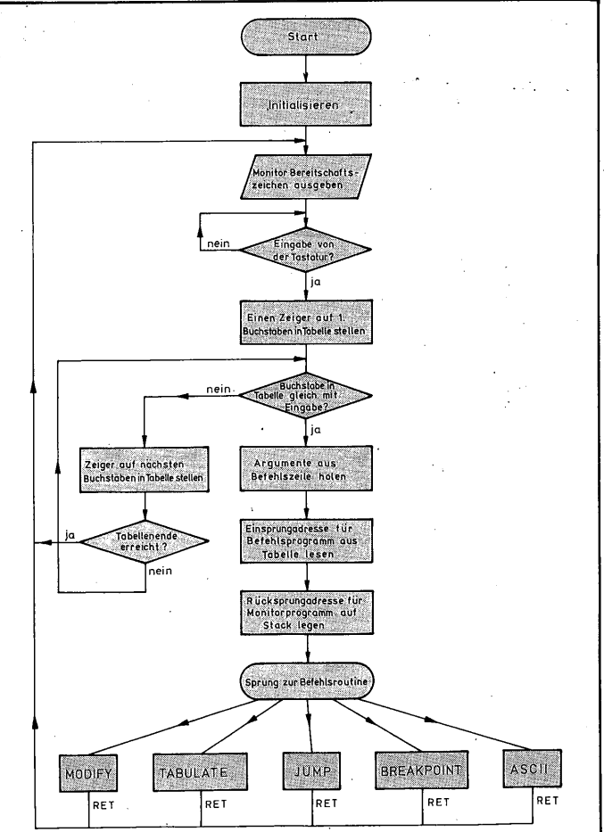
'Grobes' Flußdiagramm von MINIMON
