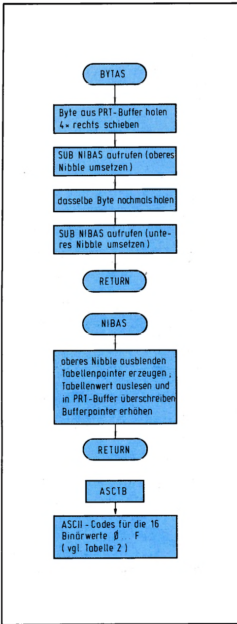
Bild 11: Zur Umsetzung eines Datenbytes in zwei ASCII-Zeichen dienen die beiden Unterprogramme BYTAS und NIBAS, die die Umsetztabelle ASCTB benutzen.
