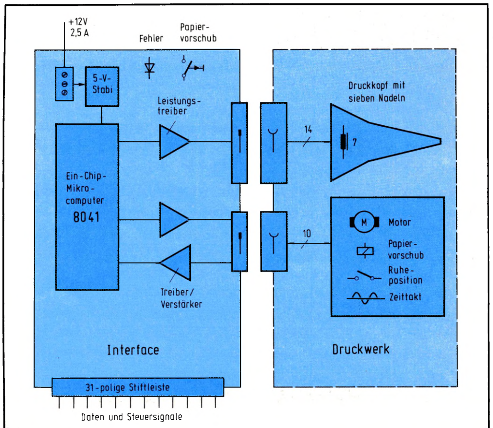
Bild 2: Die Blockschaltung zeigt, daß zur Ansteuerung des Druckwerks eine eigene Interface-Karte erforderlich ist.
