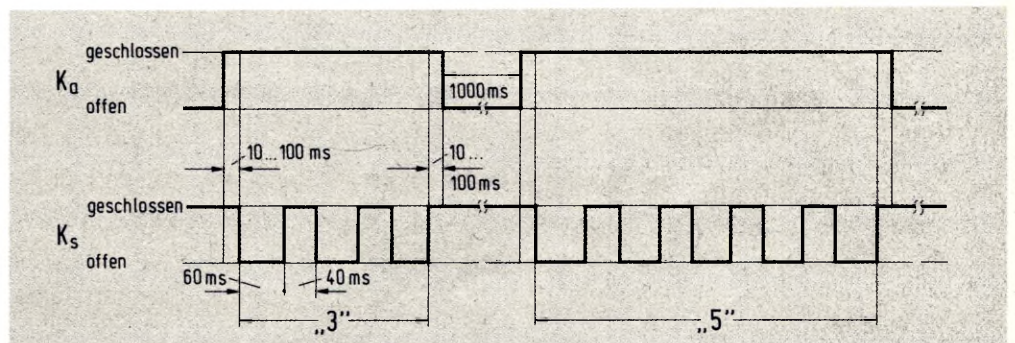
Bild 12: Ablaufdiagramm beim Wählen einer Telefon-Nummer.
