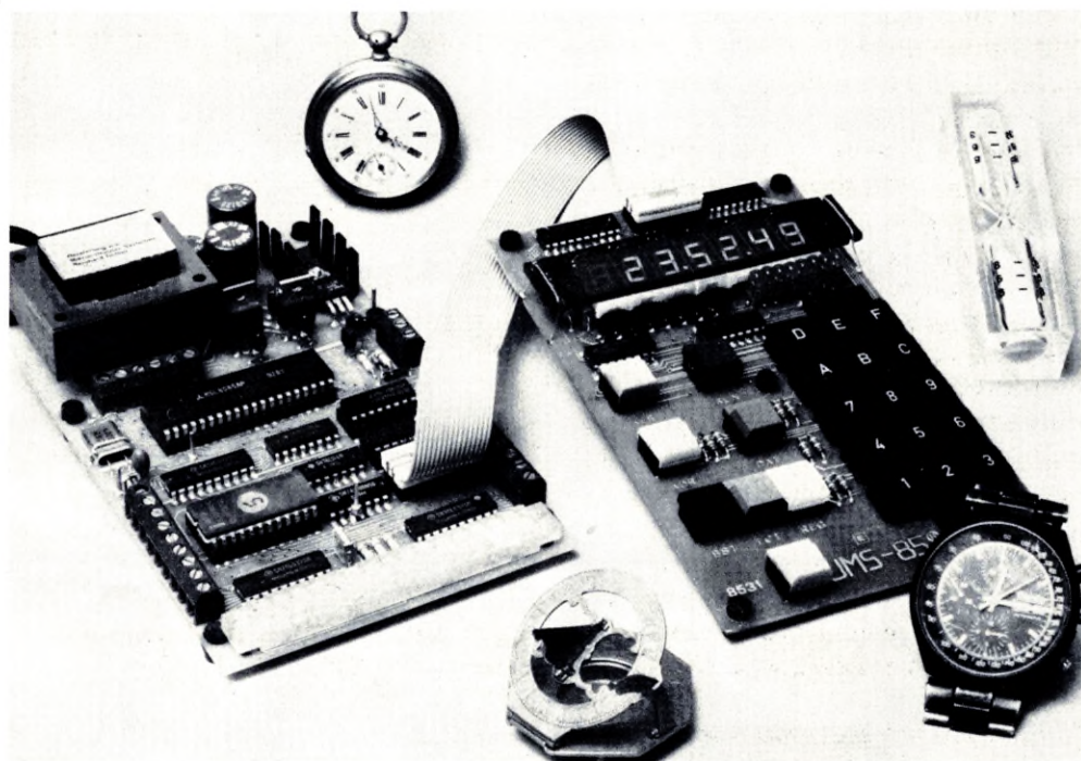
Bild 1: Bei geeigneter Programmierung wird der Mikrocomputer zur Digitaluhr – bei Bedarf sogar mit komfortabler Weckeinrichtung.
