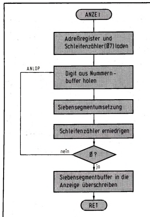
Bild 11: Vor dem Überschreiben des Siebensegmentbuffers in die Anzeige muß die Umsetzung in den Siebensegmentcode erfolgen.
