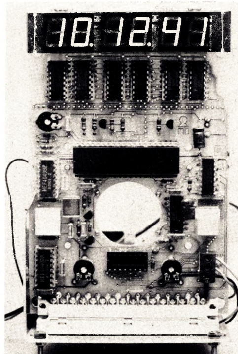
Bild 16: Die fertig bestückte Baugruppe; in der Mitte kann ein Loch herausgesägt werden, um einen Lautsprecher zentral zu befestigen.
