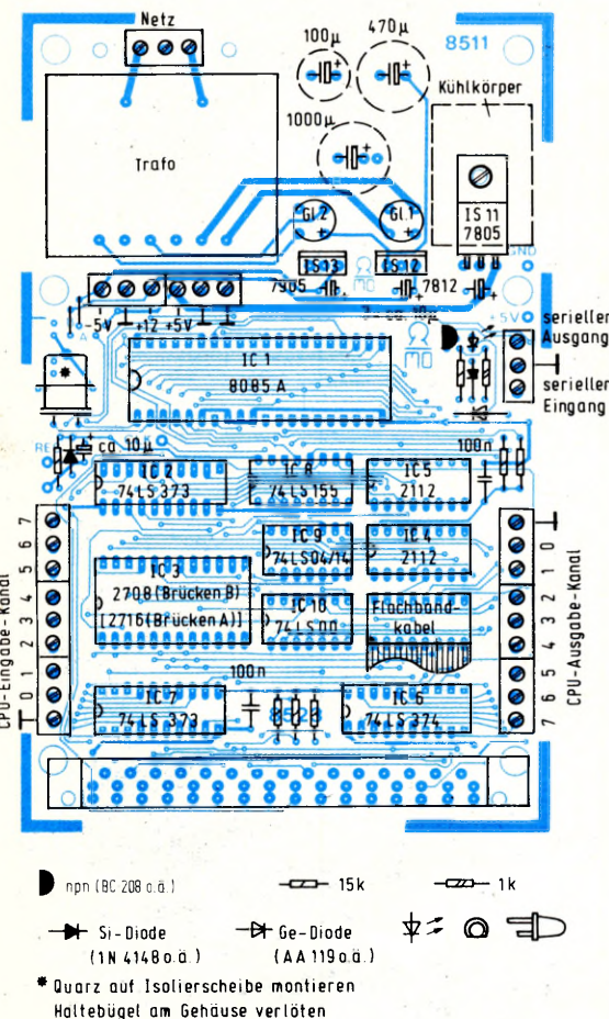
Bild 7: Bestückungsplan der Mikrocomputer-Platine mit Netzteil.
