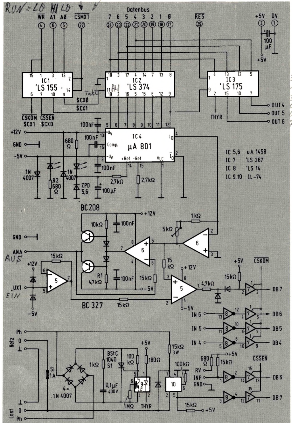
Bild 2: Das Detailschaltbild dieser Interface-Karte.
