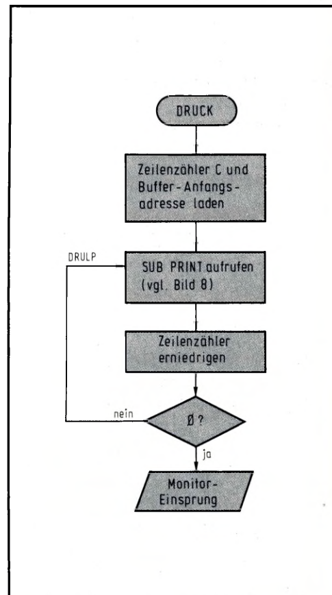
Bild 9: Mit dem übergeordneten Programm DRUCK kann man mehrere Zeilen nacheinander ausdrucken.
