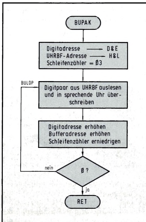
Bild 6: Mit Hilfe dieses Unterprogramms wird die Uhrzeit in die Eingangsspeicher der sprechenden Uhr überschrieben.
