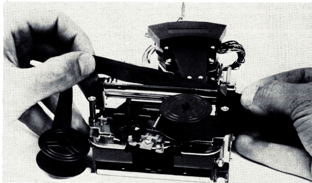
Bild 6: Beim Einsetzen des Farbbandes ist auf richtige Führung zu achten.
