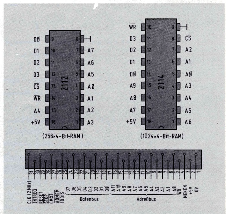
Bild 4: Zuordnung der einzelnen Adreßbits bei der UMS-RAM-Adressierung.
