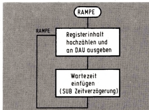
Bild 9: Ein besonders einfaches Beispiel für digital erzeugte Analogspannungen ist der Sägezahnverlauf.
