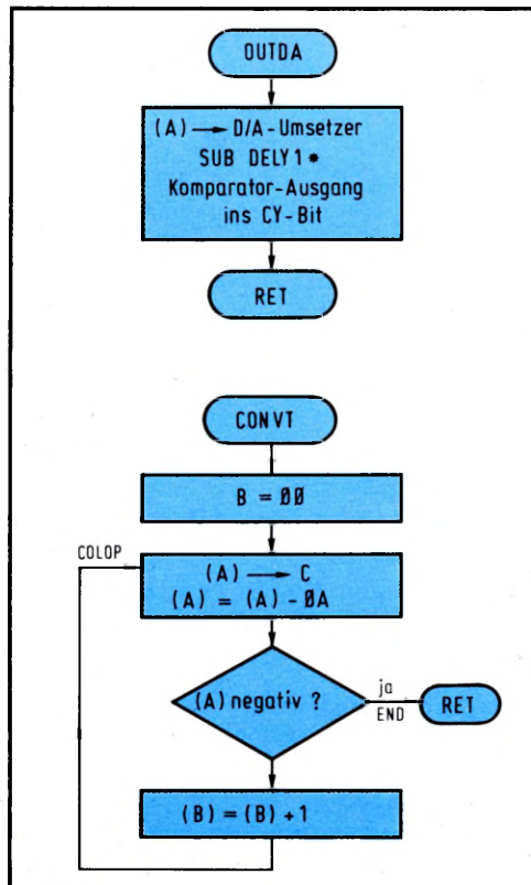
Bild 6: Zwei kleine Unterprogramme werden vom Hauptprogramm aufgerufen; OUTDA spricht den D/A-Umsetzer an, während CONVNT zur BCD-Umsetzung dient.
