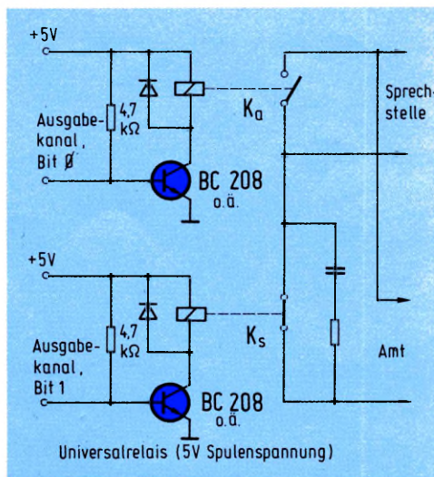
Bild 15: Die beiden Relais werden von je einem Bit des CPU-Ausgabe-Kanals angesteuert.
