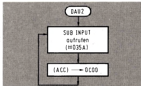
Bild 7: Mit einem UMS-85-Monitor-Programm gestaltet sich die dynamische Eingabe von Daten noch einfacher und eleganter.
