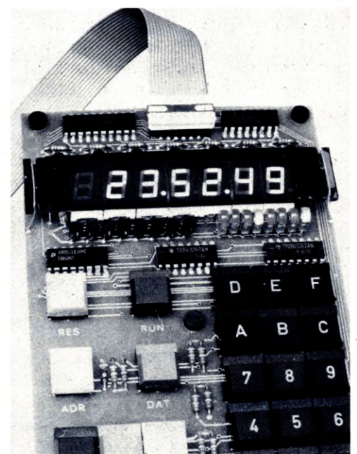
Bild 11: Die Zeit erscheint in der Anzeige und kann bei Bedarf auch Stoppuhr-Funktionen oder höhere Auflösungen liefern.
