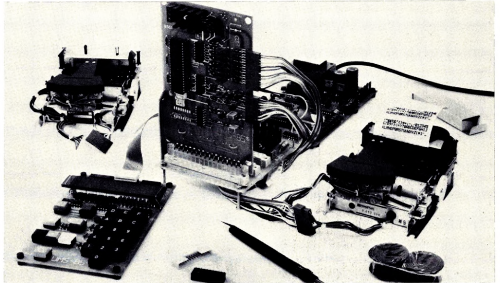
Bild 1: Mit dem Druckwerk und zugehörigem Interface wird der Mikrocomputer zum richtigen Entwicklungsplatz.
