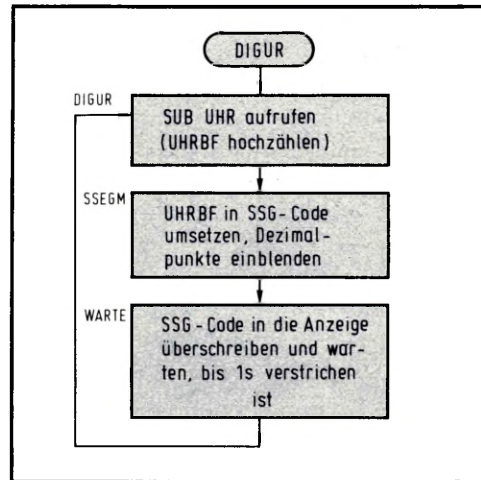
Bild 3: Das Digitaluhr-Programm besteht aus drei Aktivitäten (vgl. Bilder 4, 8 und 9).
