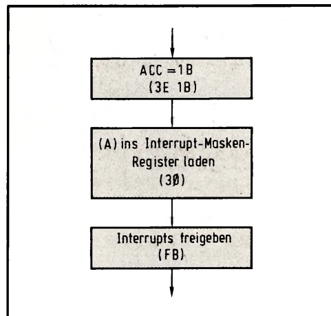
Bild 2: Bevor ein Interrupt akzeptiert werden kann, muß diese Sequenz mindestens einmal durchlaufen werden.
