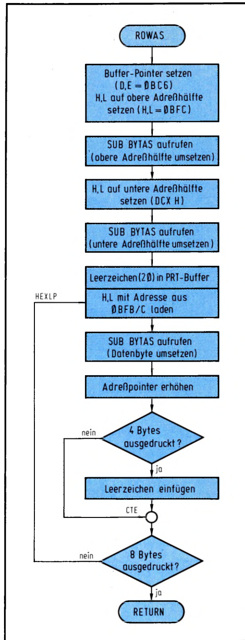
Bild 12: Unter Zuhilfenahme der Unterprogramme aus Bild 8 und 9 führt ROWAS die ASCII-Umsetzung von 8 aufeinanderfolgenden Bytes durch, denen die Anfangsadresse vorangestellt wird.
