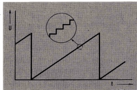
Bild 10: Bei genauem Hinsehen erkennt man, daß sich der Spannungsverlauf am DAU-Ausgang nicht stetig, sondern in winzig kleinen Stufen ändert.
