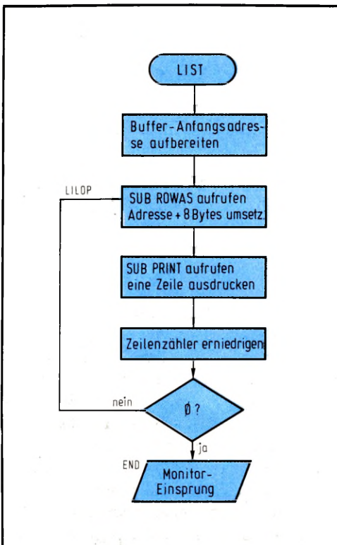
Bild 13: Das Hauptprogramm LIST kann den Speicherinhalt in hexadezimaler Form ausdrucken (vgl. Bild 15).
