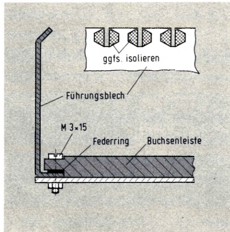
Bild 9: Wo Kurzschlußgefahr von Leiterbahnen besteht, muß das Führungsblech isoliert werden.
