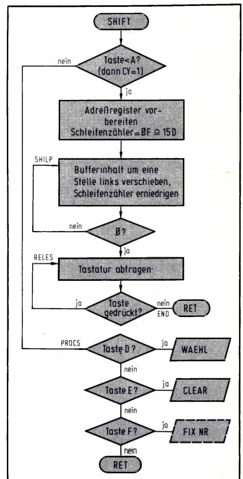
Bild 9: Bei Zifferntasten 0...9 verschiebt das Unterprogramm SHIFT den Nummernbuffer zyklisch nach links, und bei Befehlstasten verzweigt es zu den Programmteilen WAEHL bzw. CLEAR.
