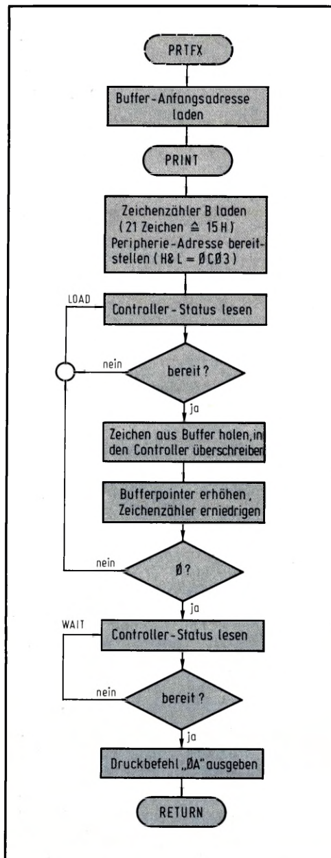
Bild 8: Unterprogramm PRINT, das 21 Zeichen aus dem RAM ausliest, in den Controller überschreibt und deren Ausdruck veranlaßt.
