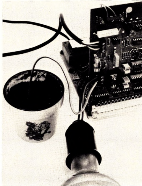
Bild 4: Last und Netz werden an die entsprechend gekennzeichneten Schraubklemmen angeschlossen.
