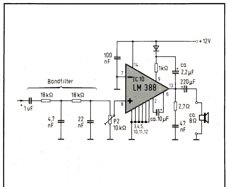
Bild 14: Ein integrierter NF-Verstärker sorgt dafür, daß die Zeitansage laut genug ertönt.
