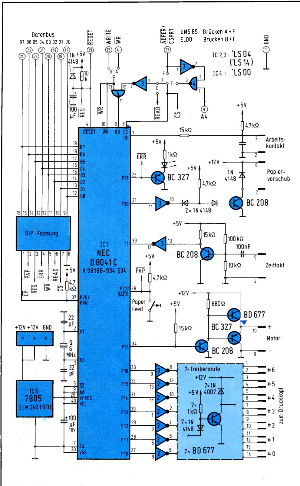
Bild 4: Die Detailschaltung der Interface-Karte.
