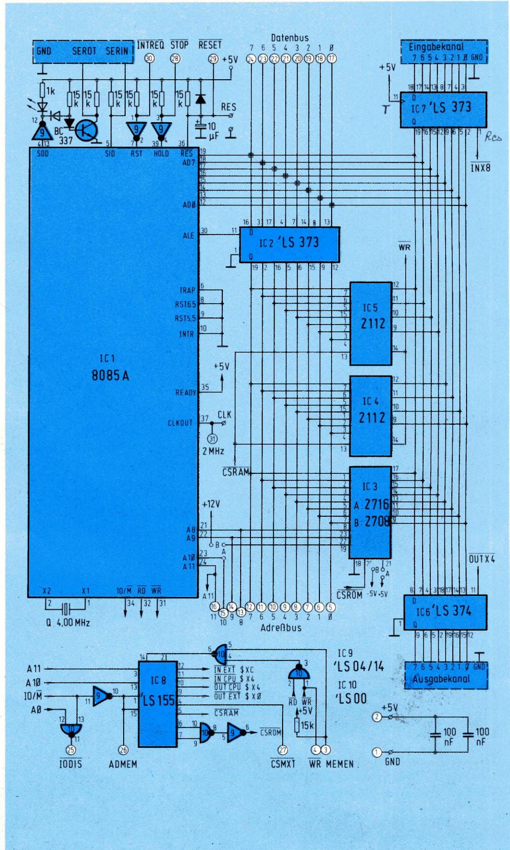
Bild 5: Schaltbild des Mikrocomputers mit Ein-/Ausgabe-Kanälen.
