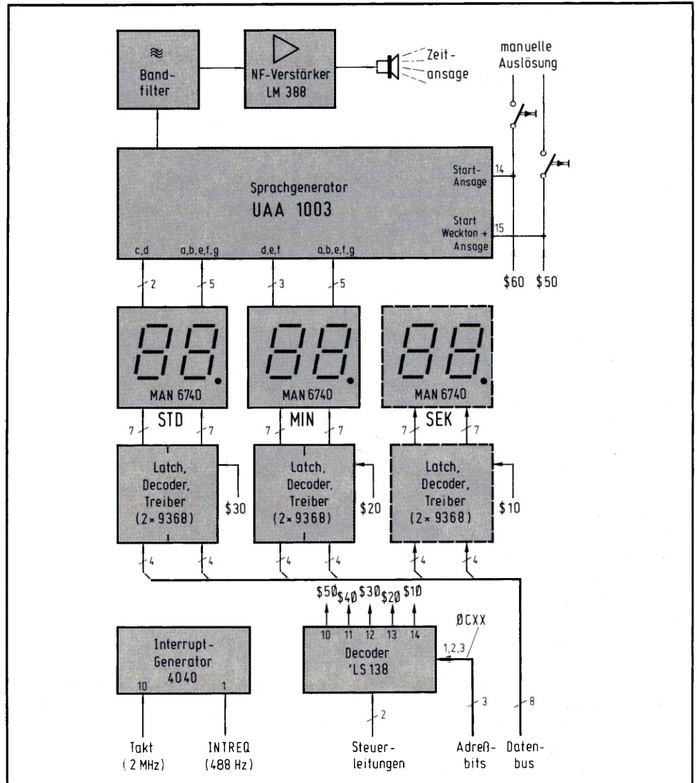
Bild 10: Blockschaltung der Interface-Karte „Sprechende Uhr“.
