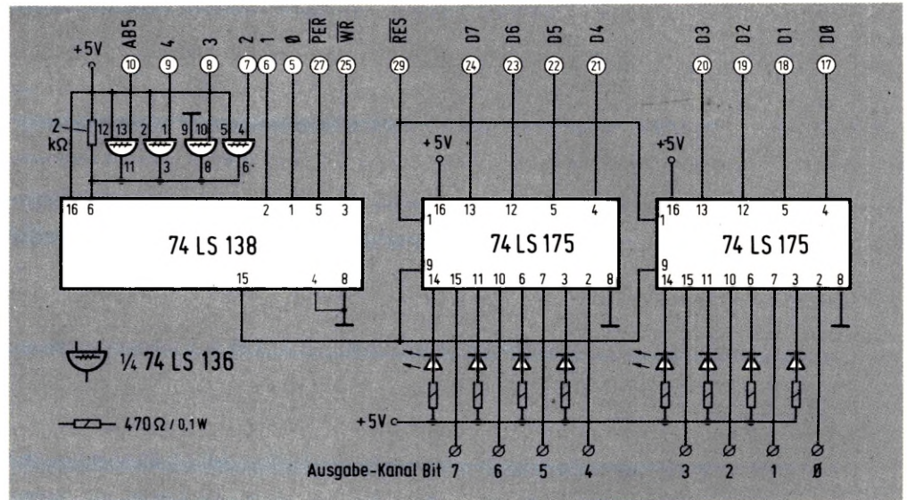
Bild 14: Ersatz des auf dem ELDO-Parallel-Interface enthaltenen Ausgabe-Kanals.
