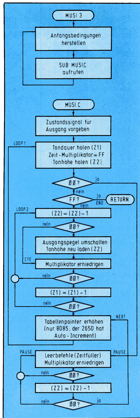
Bild 5: Das komplette Flußdiagramm für die Musikerzeugung.
