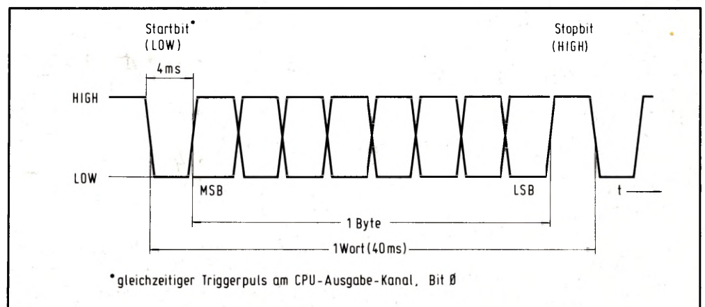
Bild 2: Bei der seriellen Datenübertragung werden pro Byte ein Start- und Stopbit ergänzt, was beim Wiedereinlesen die Synchronisation ermöglicht.
