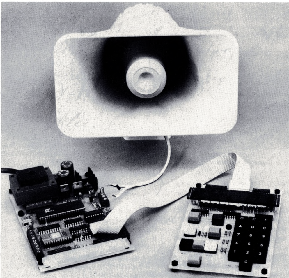
Bild 1: Ein im Monitor fest abgespeichertes Unterprogramm samt Notentabelle sorgt dafür, daß der Mikrocomputer richtige Musik erzeugen kann.
