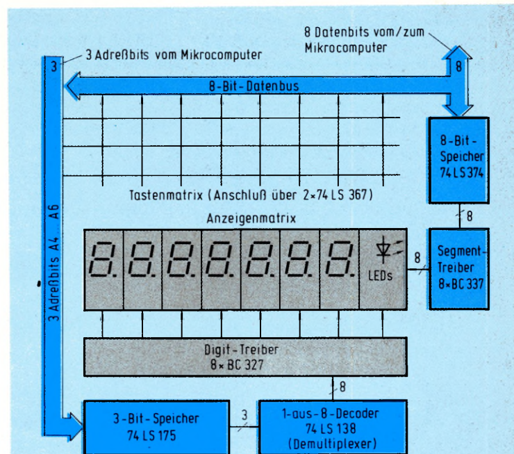
Bild 3: Blockschaltbild der Tastatur- und Anzeige-Platine.
