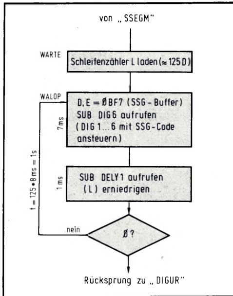
Bild 9: Während der Wartezeit wird das Unterprogramm DIG6 ständig aufgerufen, um die Anzeige dynamisch anzusteuern (softwaremäßige Erzeugung der Multiplex-Frequenz).
