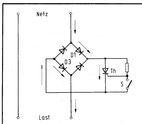
Bild 2: Als Halbleiterrelais fungiert eine Diodenbrücke mit nachgeschaltetem Thyristor, der wegen der galvanischen Trennung vom Netz über einen Optokoppler angesteuert wird.
