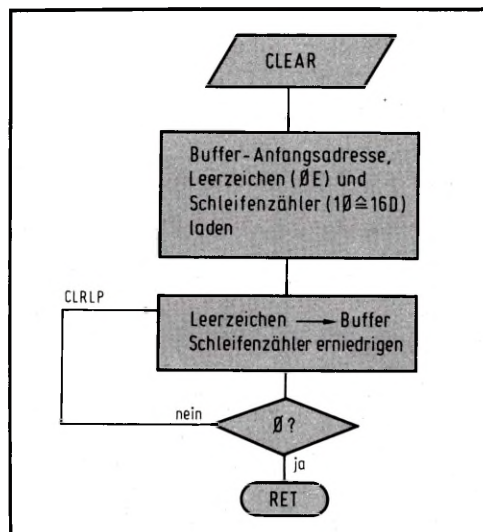
Bild 10: Programmteil CLEAR löscht den Nummernbuffer (Auffüllen mit 16 Leerzeichen 0E).
