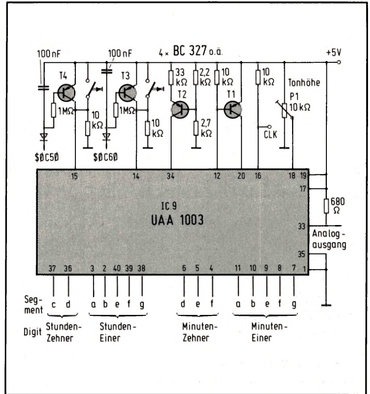
Bild 13: Beschaltung des Sprachgenerators, dessen analoges Ausgangssignal noch gefiltert und verstärkt werden muß.
