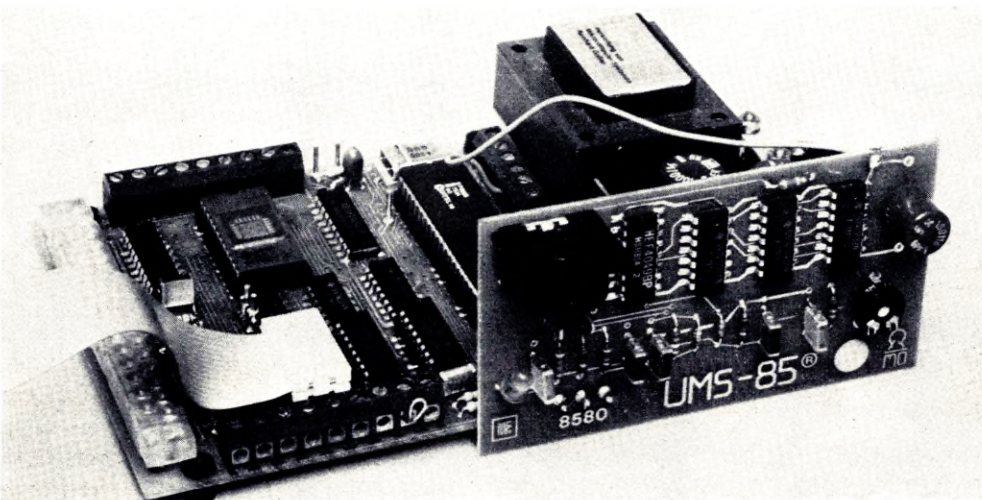
Bild 6: Die Interface-Platine wird mit drei Lötstiften in der Anschlußklemme der CPU-Karte festgeschraubt; die +5-V-Versorgung kommt über ein separates Kabel.
