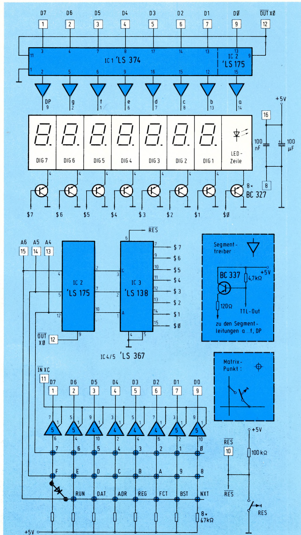
Bild 12: Bestückungsplan der Tastatur- und Anzeige-Platine.
