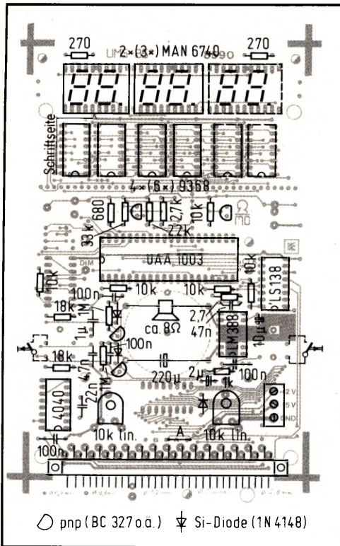
Bild 15: Bestückungsplan der sprechenden Uhr.
