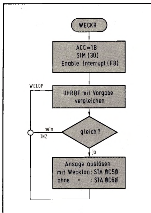
Bild 18: Programmvorschlag für einen Wecker, der die Weckzeit ansagen kann.
