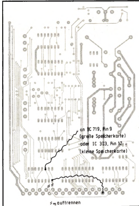
Bild 4: Für den Betrieb am ELDO müssen die gezeigten Modifikationen auf der Rückseite der Interface-Karte durchgeführt werden.
