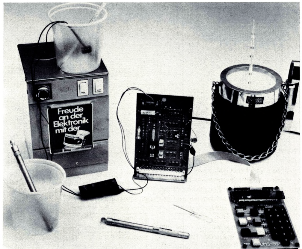
Bild 1: Mit einer simplen Siliziumdiode als Sensor arbeitet das Digitalthermometer, dessen Realisierung dieser Beitrag beschreibt.
