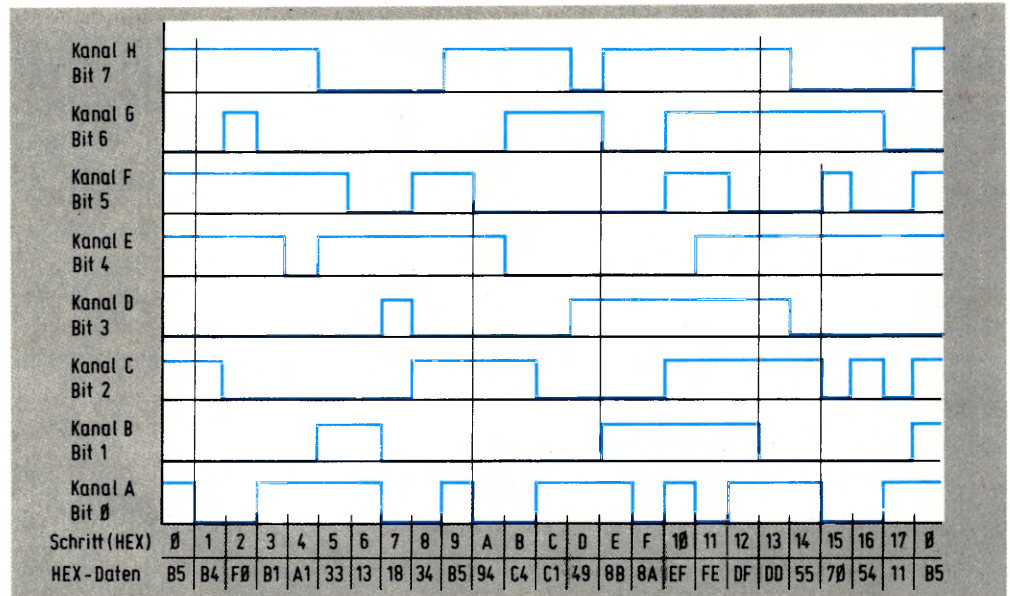
Bild 12: Beispiel einer achtkanaligen Ablaufsteuerung.
