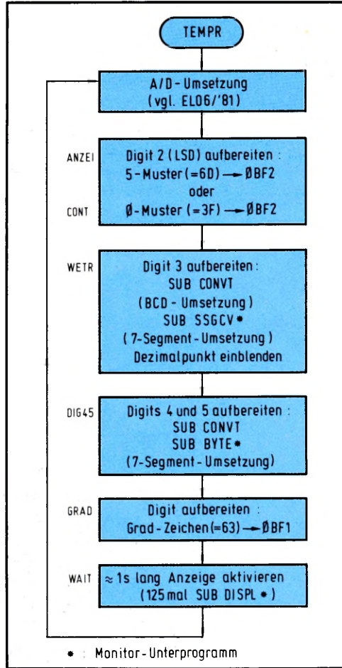
Bild 5: Im wesentlichen weist das Hauptprogramm TEMPR eine lineare Struktur auf.
