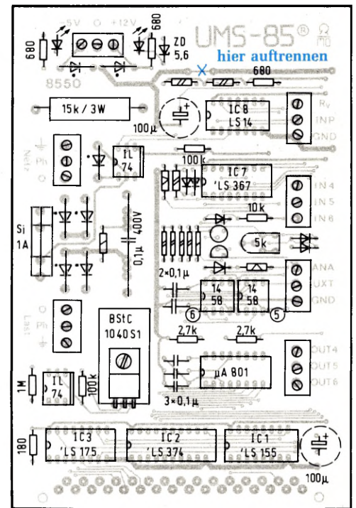
Bild 4: Mit der Trennung von digitaler und analoger Masse erreicht man eine verbesserte Störspannungsunterdrückung.
