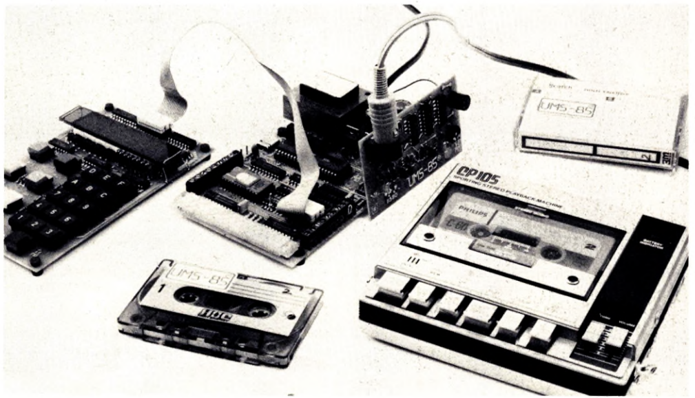
Bild 1: Mit dem Cassetten-Interface können handelsübliche Recorder als externer Massenspeicher benutzt werden.
