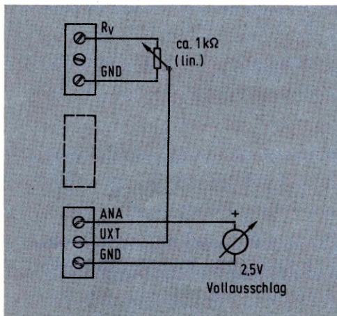
Bild 12: Der Poti-Abgriff simuliert eine zu messende Spannung; Sie können natürlich auch z. B. eine Batterie anschließen.
