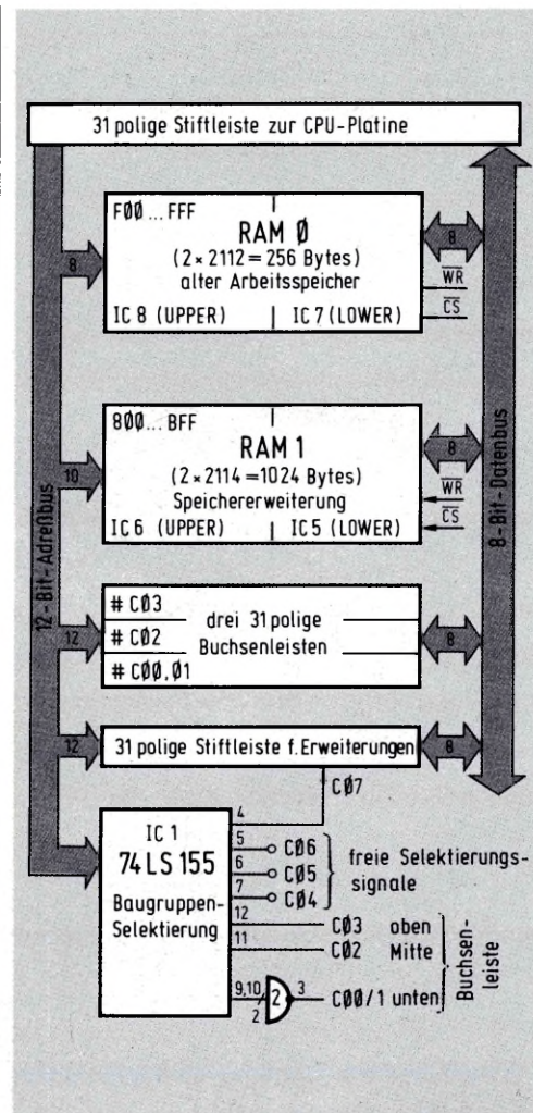
Bild 3: Das Blockschaltbild zeigt den Aufbau der Erweiterungskarte.
