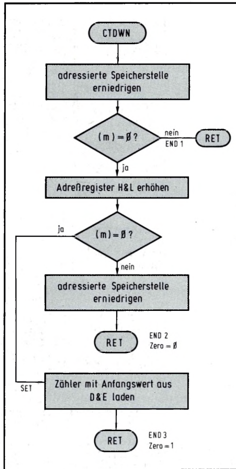
Bild 5: SUB Countdown erniedrigt einen 16-Bit-Zähler (gebildet aus zwei Bytes im RAM) und setzt beim Nullzustand das Zero-FLAG.
