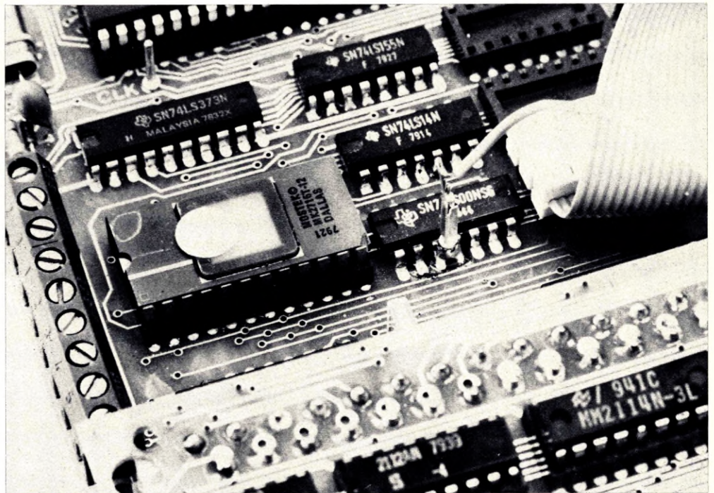
Bild 10: Eine separate Steckverbindung führt der Erweiterungskarte das CS-Signal zu.
