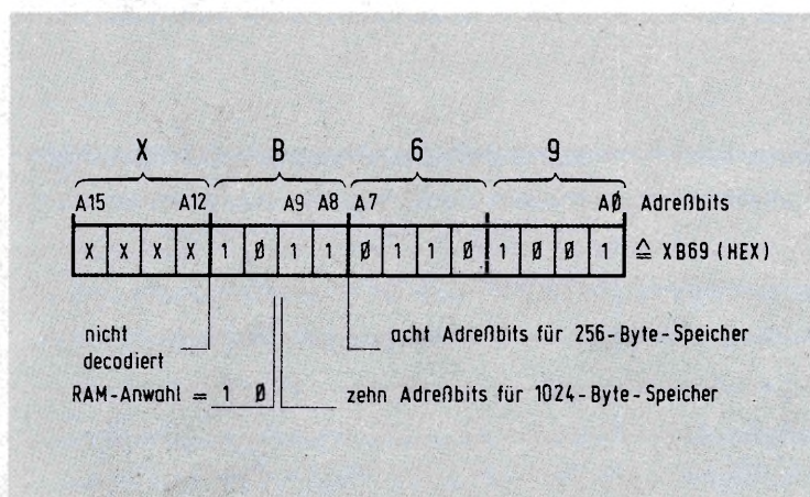
Bild 4: Zuordnung der einzelnen Adreßbits bei der UMS-RAM-Adressierung.
