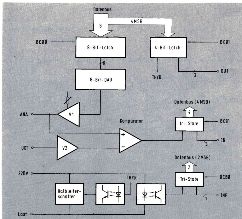
Bild 1: Aus der Blockschaltung sind die einzelnen Funktionseinheiten zu erkennen.
