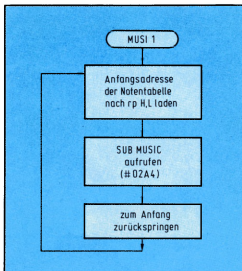
Bild 2: Der Aufruf des MUSIC -Unterprogramms erfordert nur drei Aktivitäten.
