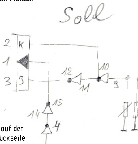
Bild 4: Bestückungsplan der nur 100 x 55 mm 2 großen Platine.
