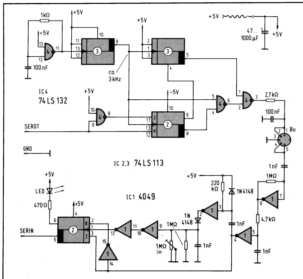
Bild 3: Schaltung des Cassetten-Interfaces.
