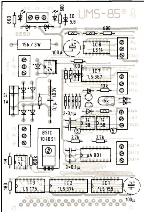
Bild 3: Der Bestückungsplan zeigt die übersichtliche Anordnung der Bauteile.
