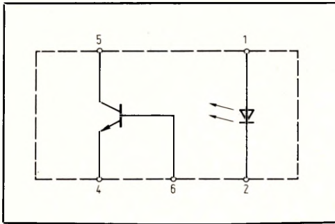
Bild 3: Die Informationsübertragung in einem Optokoppler erfolgt kontakt- und berührungslos mittels Licht.
