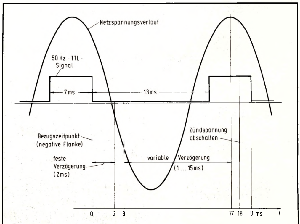
Bild 5: Über einen zweiten Optokoppler wird ein netzspannungssynchrones TTL-Signal bereitgestellt.
