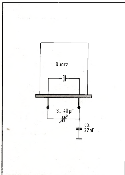
Bild 17: Mit dieser Kondensator-Beschaltung läßt sich der Quarzoszillator des 8085 exakt abgleichen.
