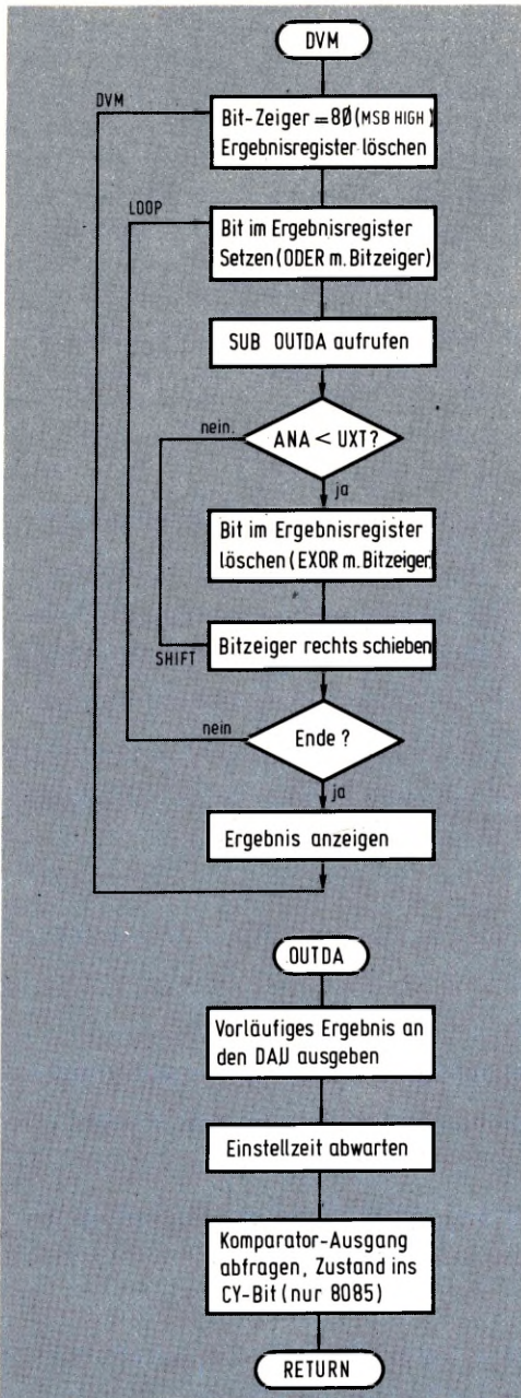
Bild 11: Dieses einfache Programmbeispiel macht aus dem Mikrocomputer samt Analog-Interface ein funktionierendes Digitalvoltmeter.
