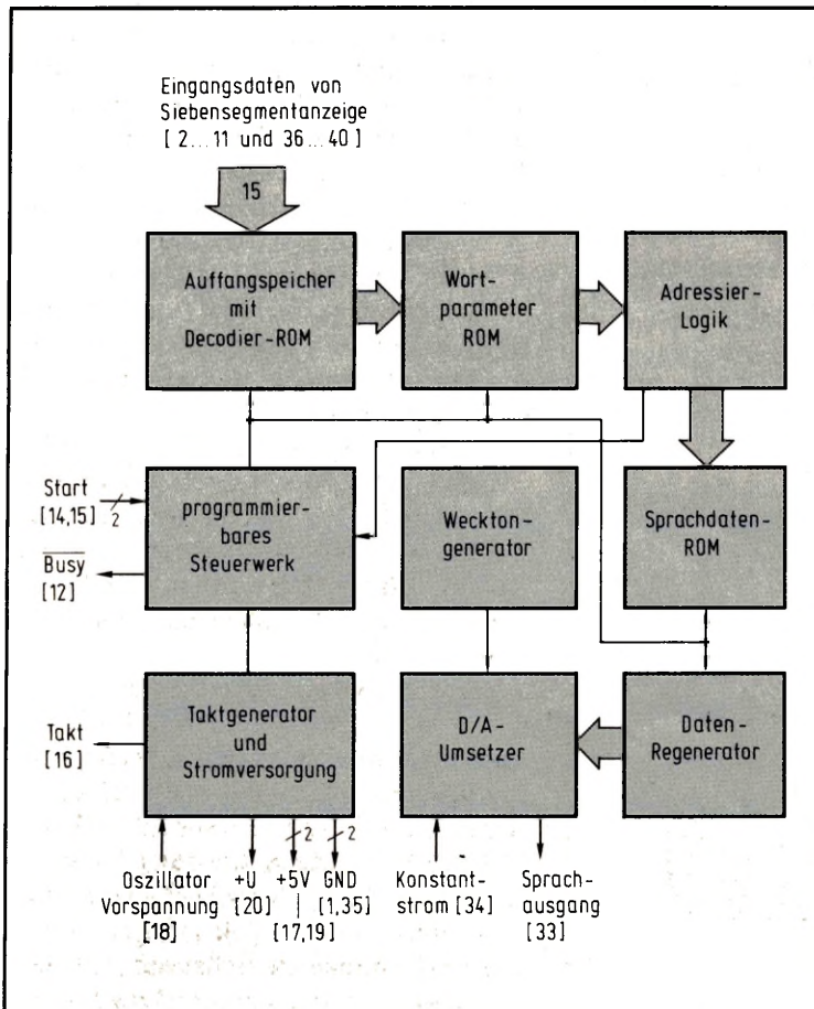
Bild 12: Interner Aufbau des Sprachgenerators UAA 1003.
