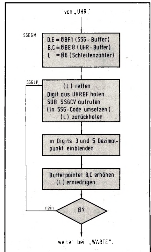
Bild 8: Die Siebensegmentumsetzung der sechs Zähler vollzieht sich über den Aufruf von SSGCV.
