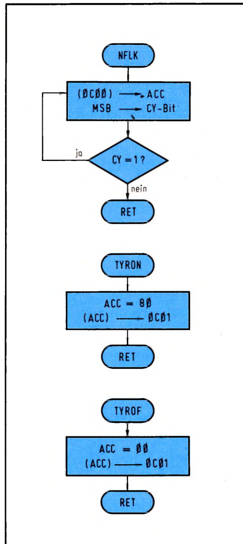
Bild 7: Das Hauptprogramm verwendet drei kleine Unterprogramme zur Flankenerkennung (NFLK) sowie zum Ein- und Ausschalten des Thyristors (TYRON bzw. TYROF).
