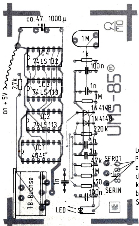
Bild 4: Bestückungsplan der nur 100 x 55 mm 2 großen Platine.
