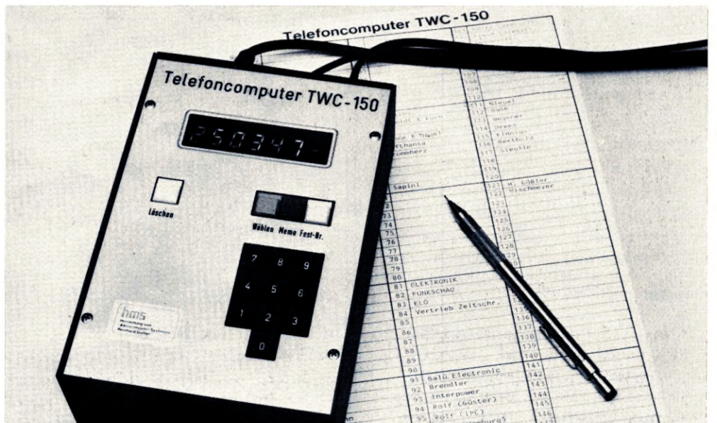
Bild 13: Entwicklungsstudie für einen automatischen Rufnummernspeicher und -geber auf der Basis des UMS-85, der bis zu 150 Festnummern auf Abruf bereithalten kann.
