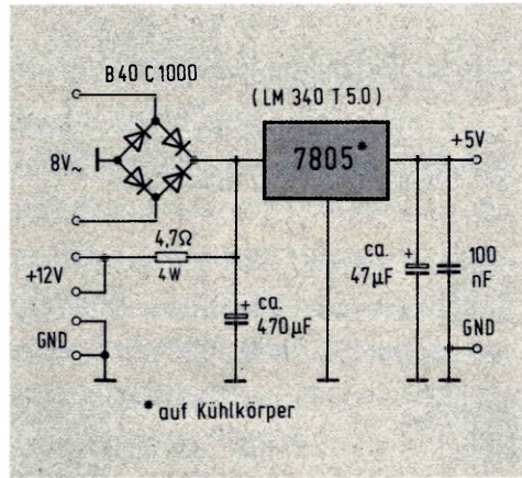
Bild 6: Auf der Erweiterungskarte ist ein eigener Festspannungsregler zur Stromversorgung vorgesehen.
