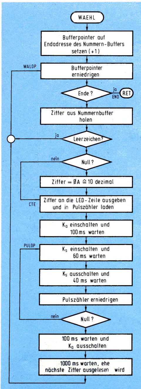
Bild 13: Flußdiagramm für ein Unterprogramm, das Telefon-Nummern „wählen“ kann.
