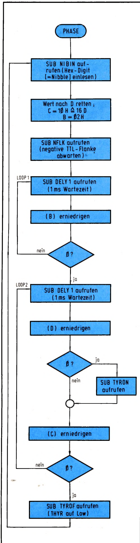
Bild 6: Flußdiagramm für das Programm der Phasenanschnittsteuerung.
