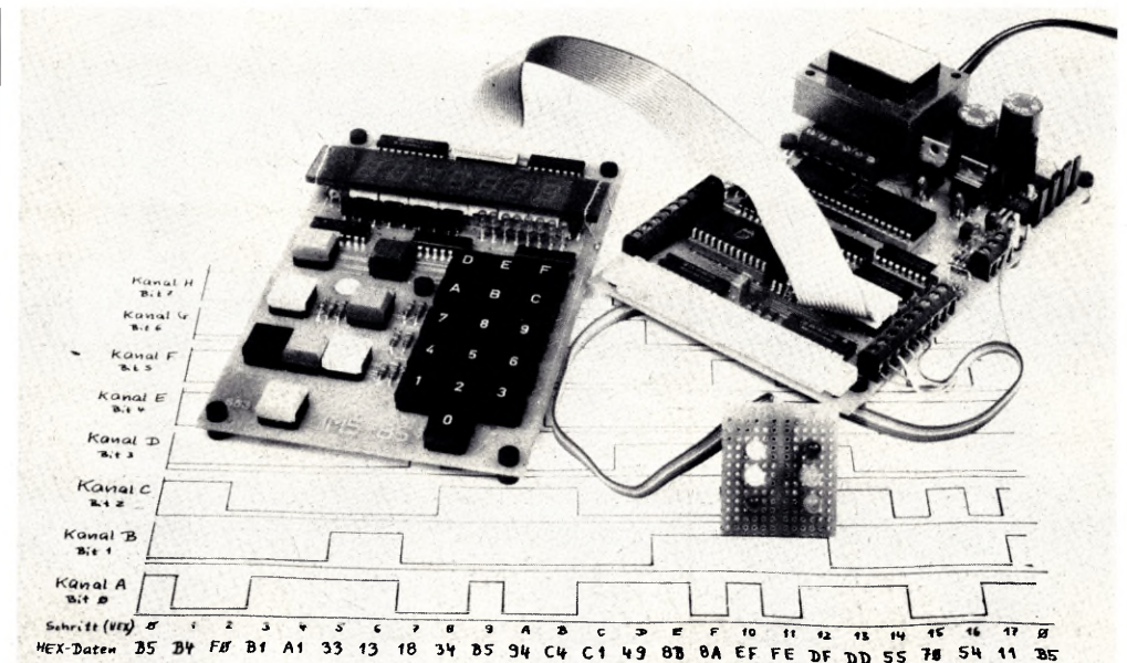
Bild 1: Schon mit geringem Aufwand kann man einen Mikrocomputer zum programmierbaren Schaltwerk machen.
