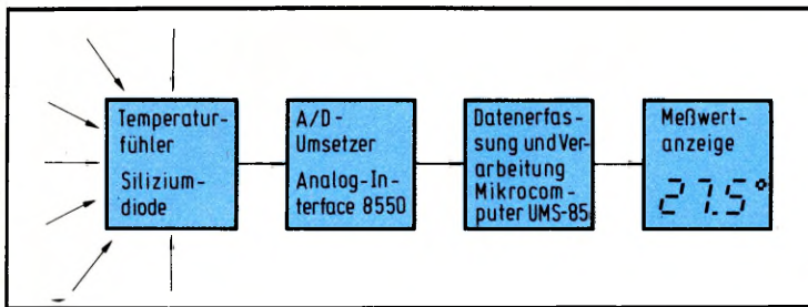
Bild 2: Blockschaltung des Thermometers auf Mikrocomputer-Basis.
