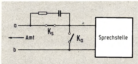
Bild 11: Zwei Kontakte, ein Öffner und ein Schließer, übernehmen das „Wählen“ der gewünschten Nummer.
