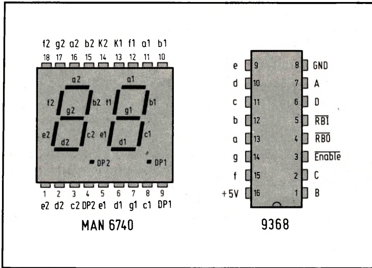
Bild 11: Der Decoder 9368 besitzt einen 4-Bit-Eingangsspeicher; seine Ausgänge treiben die Segmente direkt ohne Vorwiderstände.
