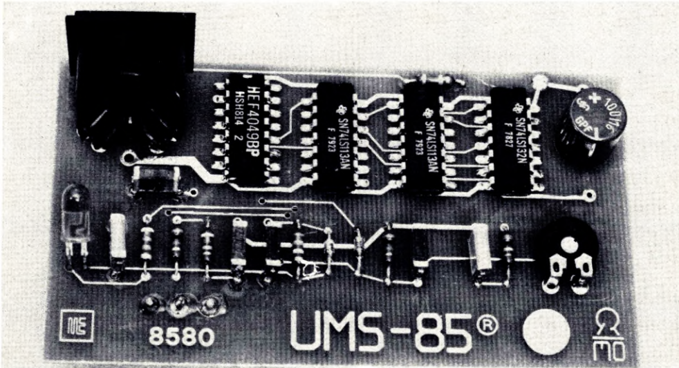
Bild 5: Ansicht des fertig bestückten Cassetten-Interfaces.
