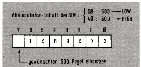
Bild 10: Beeinflussung des SOD-Ausgangs am 8085.
