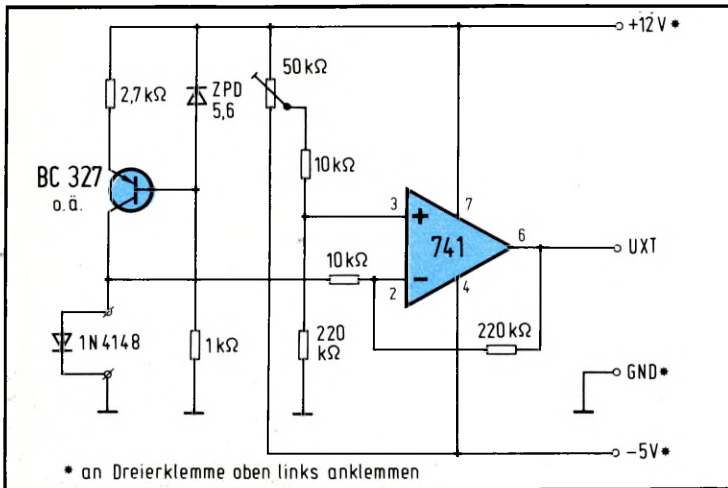
Bild 3: Konstantstromquelle und Operationsverstärker bereiten das von der Diode gelieferte Signal auf.
