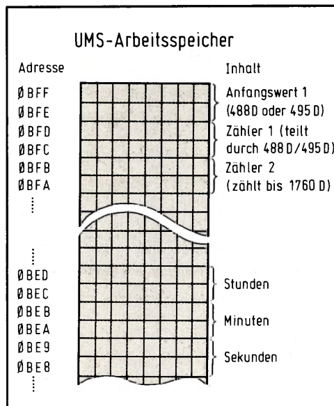
Bild 3: Die softwaremäßige Teilung der eingespeisten Interrupt-Frequenz erfordert noch einmal sechs RAM-Zellen.
