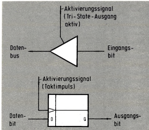
Bild 2: Tri-State-Gatter und D-Flipflop ersetzen in einfachen Anwendungen komplexe Peripheriebausteine.
