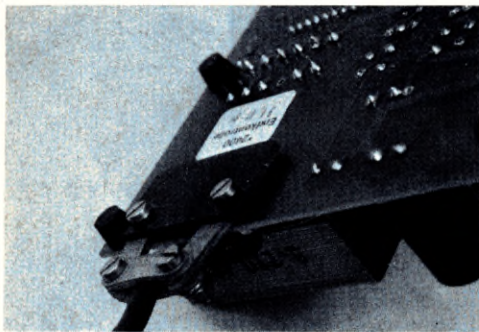
Bild 10: Das fertig montierte Netzkabel mit Zugentlastung und Berührungsschutz.
