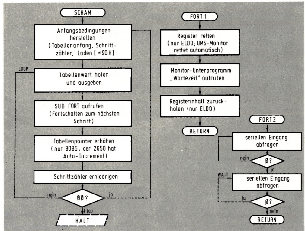
Bild 13: Flußdiagramm für das Programmbeispiel „Schaltautomat“.
