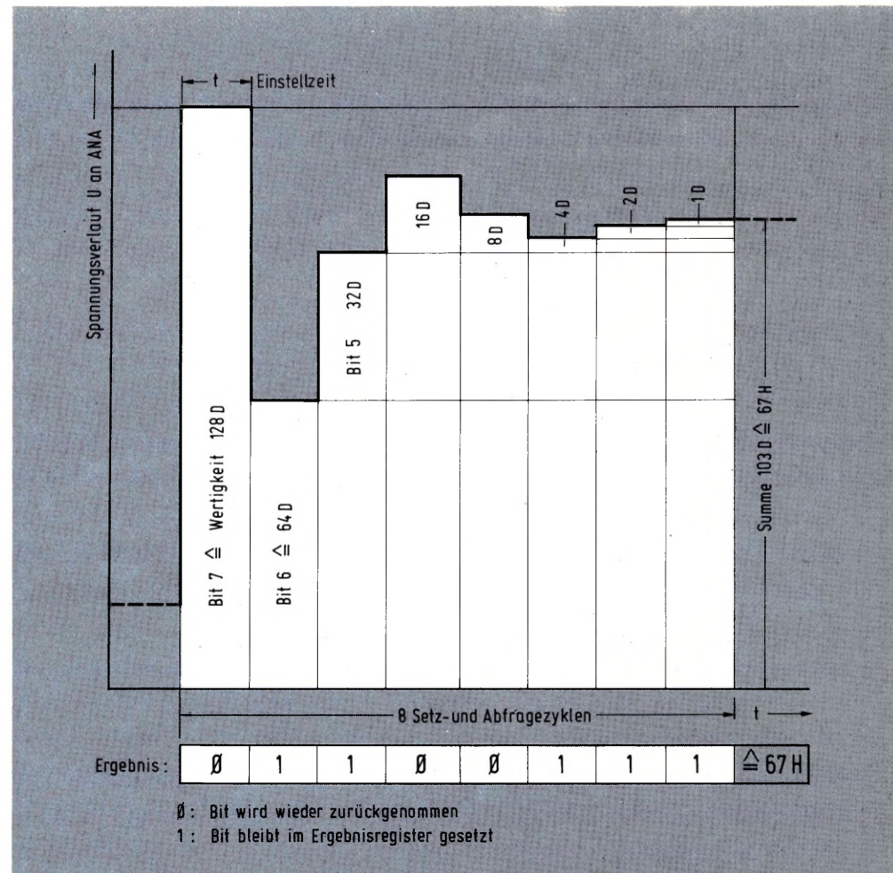
Bild 14: Diese Grafik verdeutlicht die Vorgehensweise bei der schrittweisen Annäherung an den Endwert.
