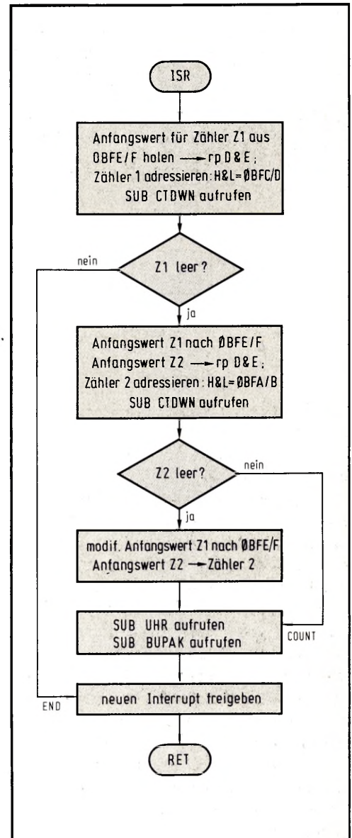
Bild 4: Die Interrupt-Service-Routine sorgt dafür, daß das Hochzählen des Uhrzeit-Buffers nur einmal pro Sekunde erfolgt.
