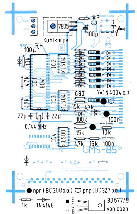
Bild 5: Auf dem Bestückungsplan ist die übersichtliche Anordnung der Bauteile zu erkennen.
