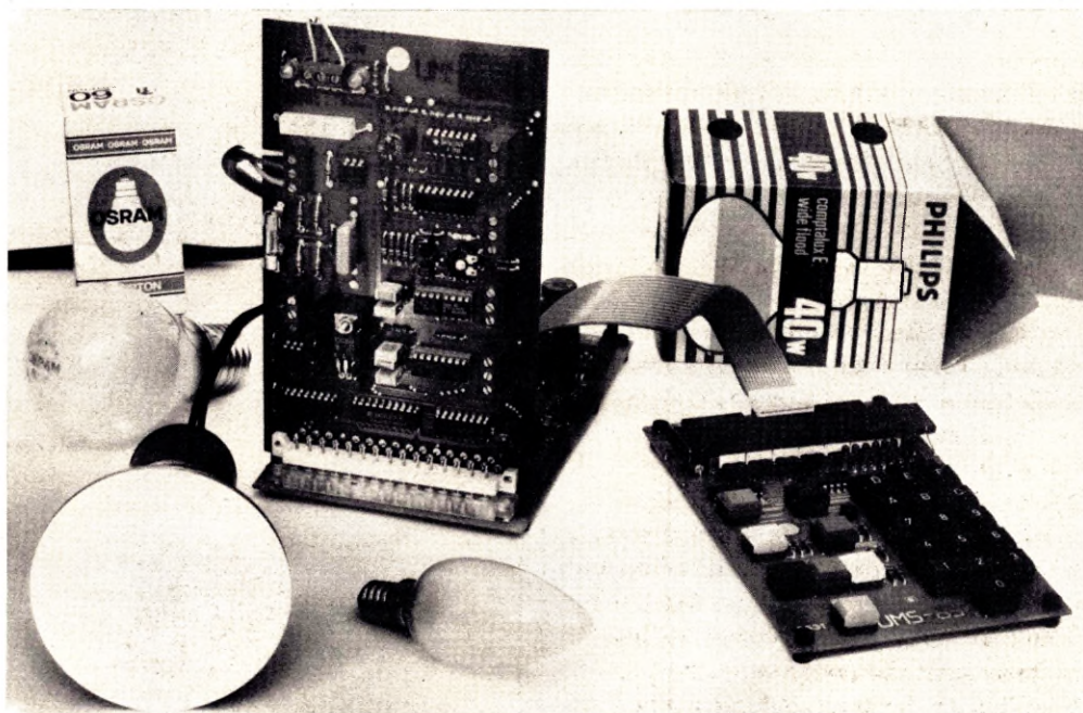
Bild 1: Über einen kontaktlosen Halbleiterschalter besteht sogar die Möglichkeit, Lasten im 220-V-Netz zu schalten.
