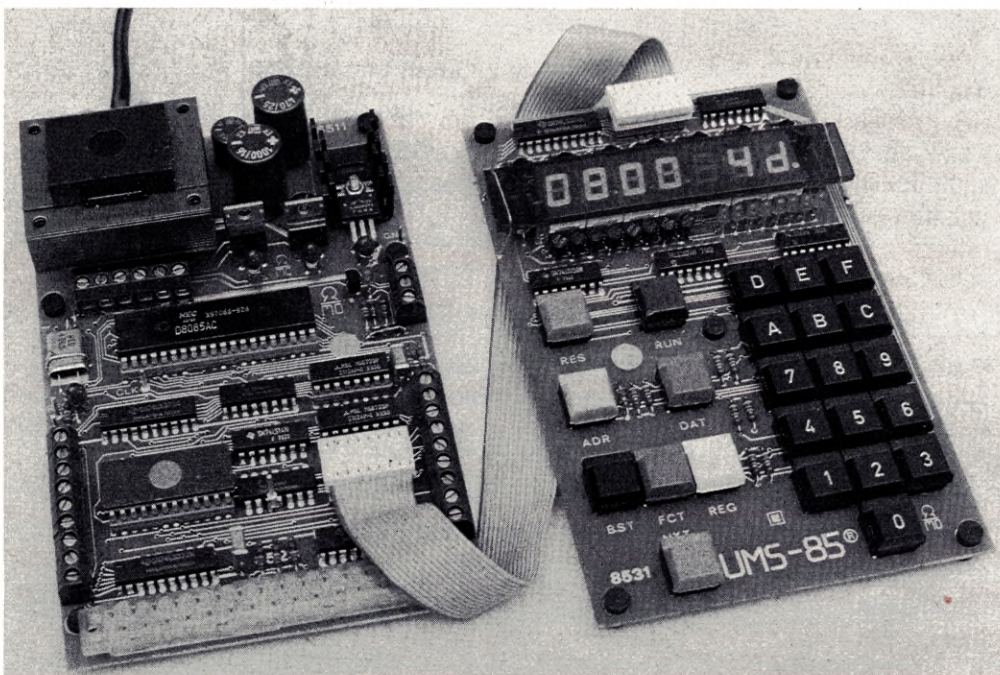
Bild 1: Auf Standard-Europakarten sind Mikrocomputer sowie Tastatur und Anzeige untergebracht.
