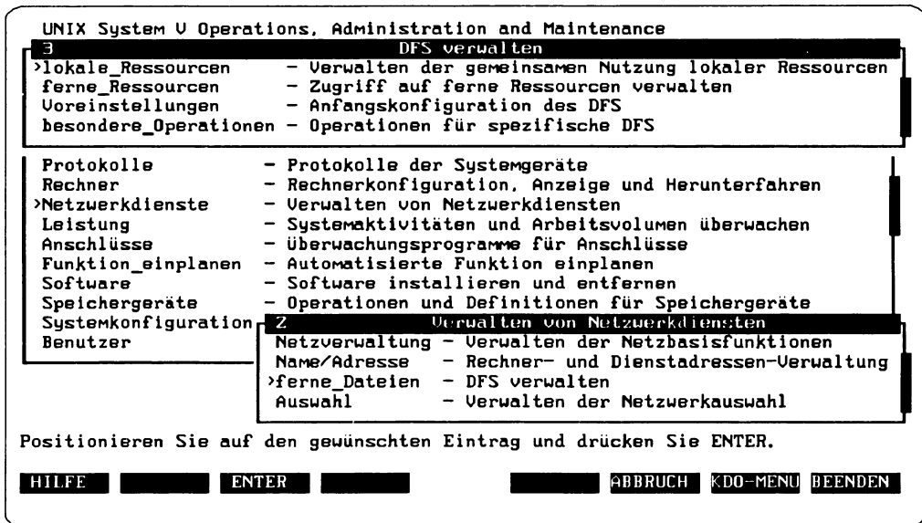
Abbildung 4: NFS verwalten
